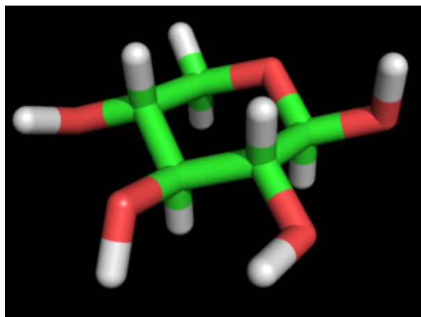
Xylopyranose ?-D
