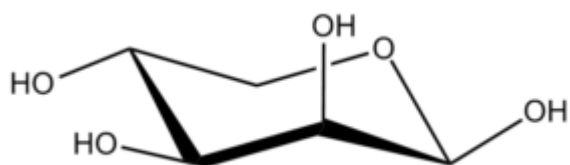
Lyxopyranose ?-D
