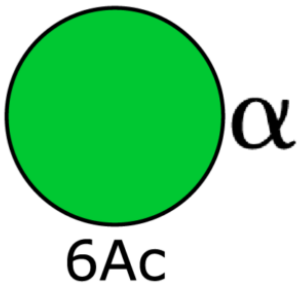
Mannopyranose 6OAc ?-D
