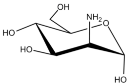
Mannosamine \beta -D
