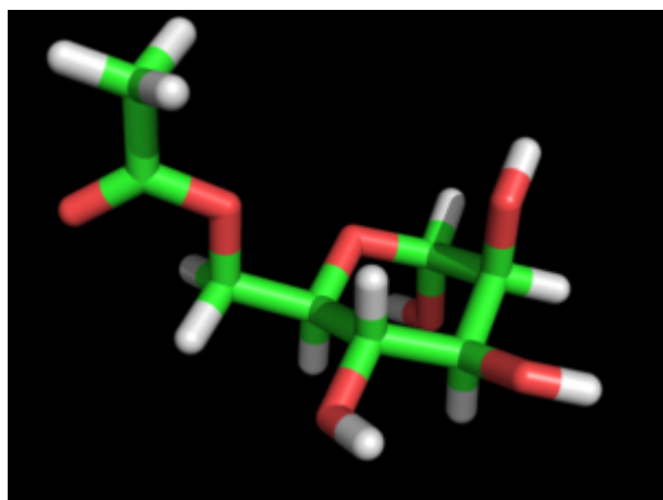
Mannopyranose 6OAc ?-D
