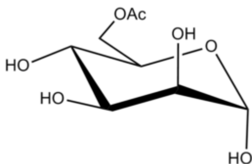
Mannopyranose 6OAc ?-D
