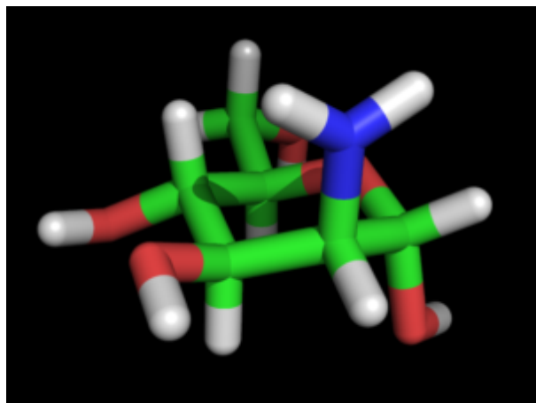
Mannosamine \beta -D
