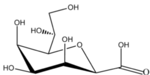
Ko : L-glycero-D-Talo-oct-2-ulosonic Acid
