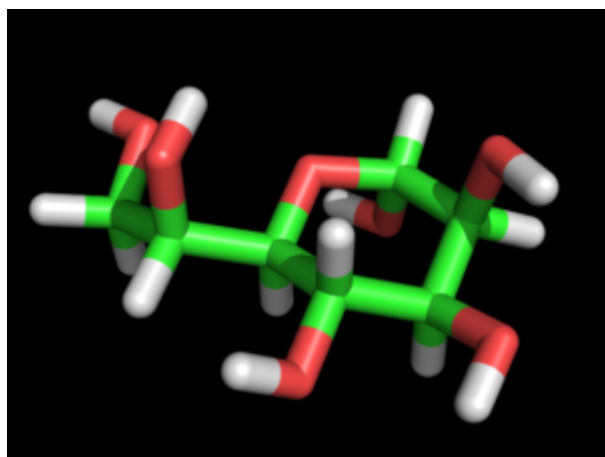
D-Heptose ?-D
