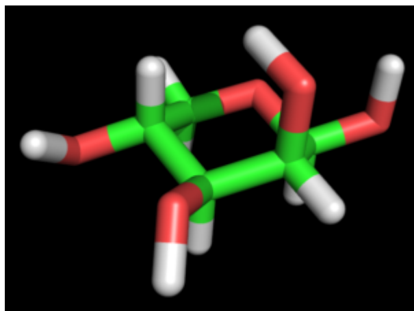
Lyxopyranose ?-D
