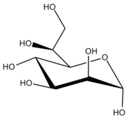
D-Heptose ?-D
