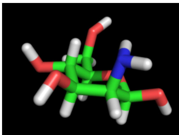
Mannosamine ?-D
