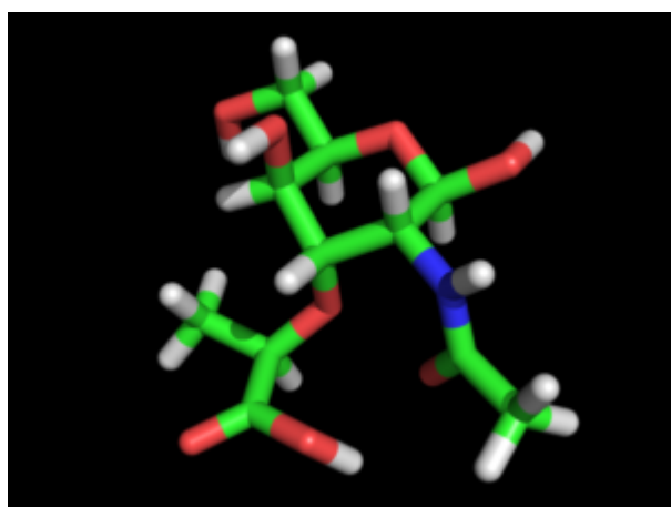
MurNAc ?-D
