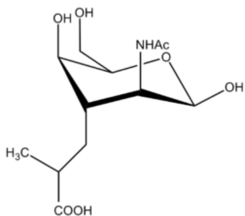
MurNAc ?-D
