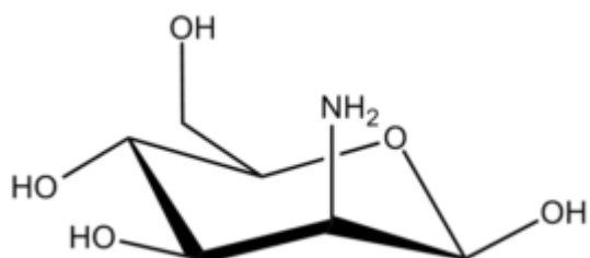
Mannosamine ?-D
