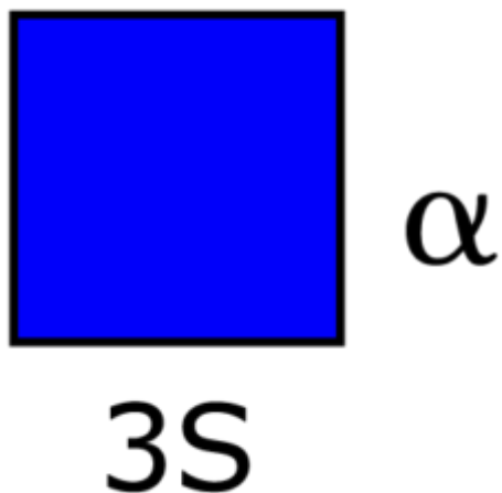
Glucosamine 3-S ?-D
