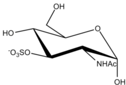
Glucosamine 3-S ?-D
