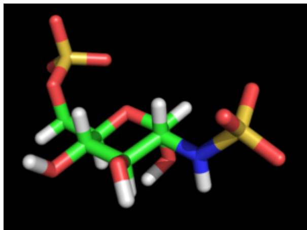
Glucosamine 6-S ?-D
