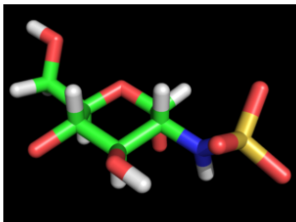
Glucosamine NS Î±-D
