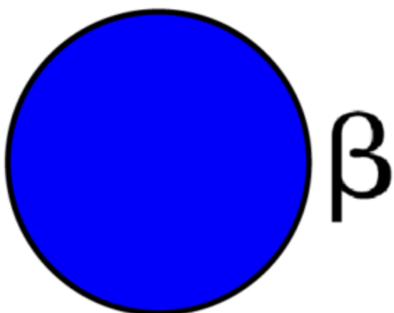
Glucopyranose ?-D
