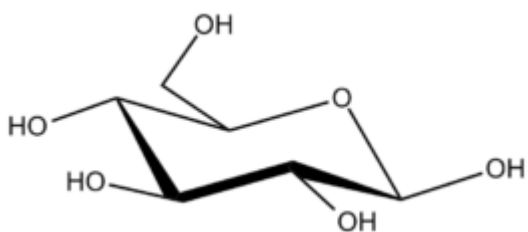
Glucopyranose ?-D
