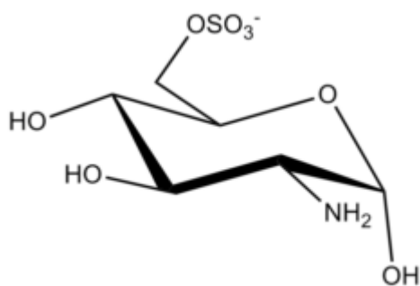
Glucosamine 6-S ?-D
