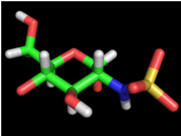
Glucosamine NS \alpha -D
