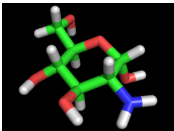
Glucosamine ?-D
