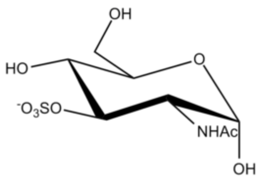
Glucosamine 3-S Î±-D
