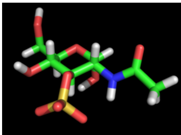
Glucosamine 3-S ?-D
