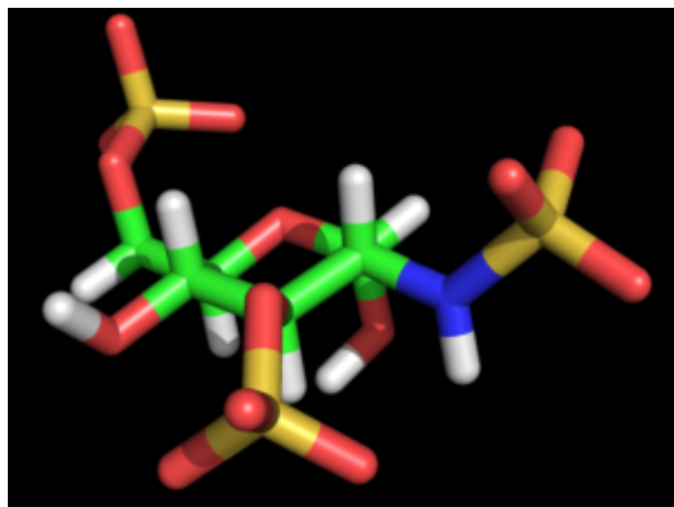
Glucosamine NS 3,6-S ?-D
