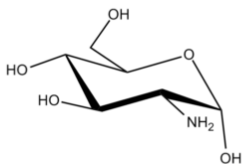
Glucosamine ?-D
