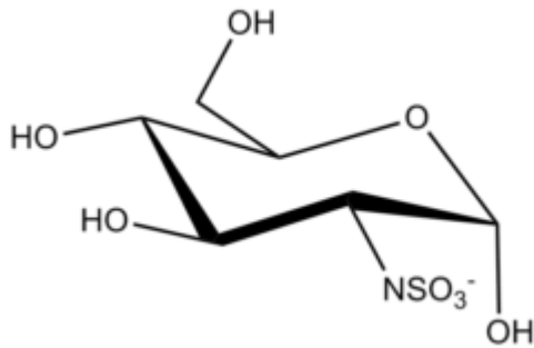
Glucosamine NS \alpha -D
