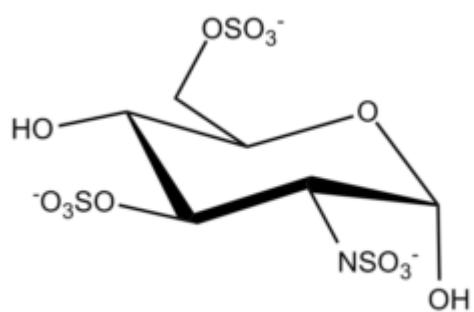
Glucosamine NS 3,6-S ?-D
