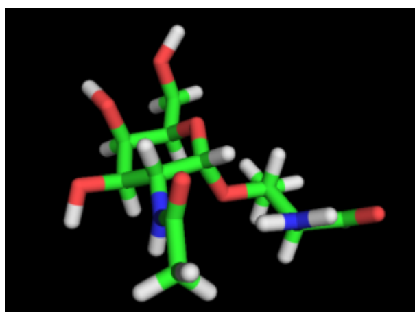
\beta -D 1-3 Thr
