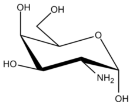
Galactosamine ?-D
