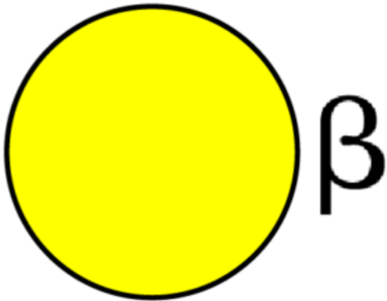
Galactopyranose ?-D
