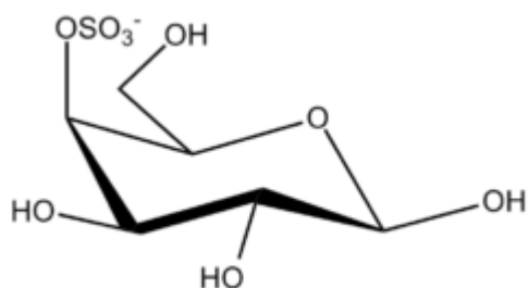
32b. Galactopyranose 4-Sulfate \hat{1}^2 -D
