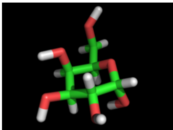
Galactopyranose ?-D
