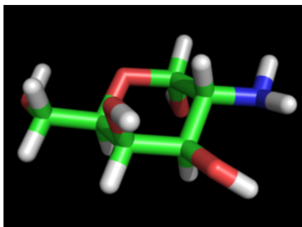
Galactosamine ?-D
