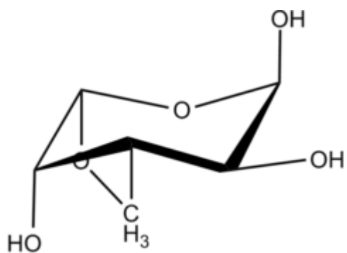
Galactopyranose 3,6 anhydro ?-L
