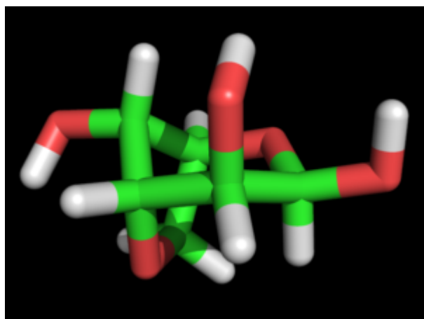
Galactopyranose 3,6 anhydro ?-L
