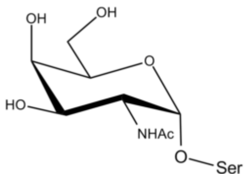
N-Acetyl Galactosamine ?-D 1-3 Ser
