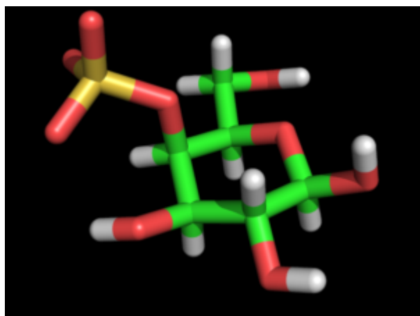
32c. Galactopyranose 4-Sulfate \hat{1}^2 -D
