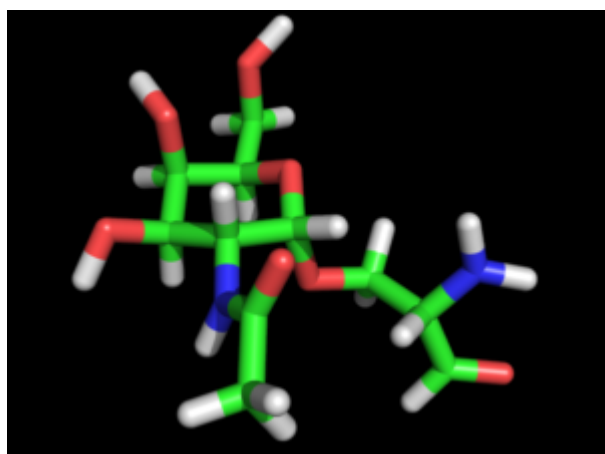
N-Acetyl Galactosamine ?-D 1-3 Ser
