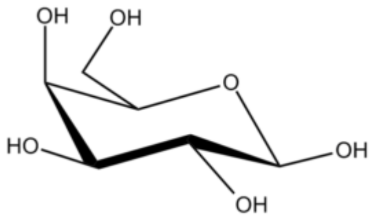
Galactopyranose ?-D
