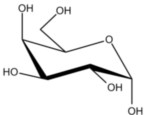
Galactopyranose ?-D
