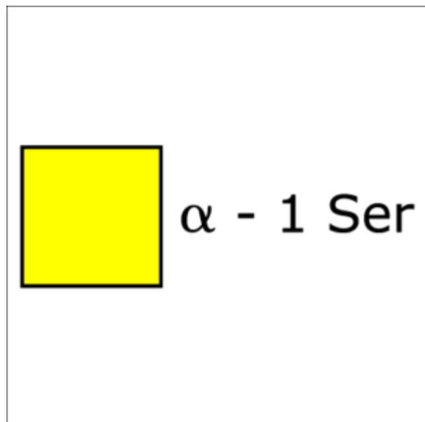
N-Acetyl Galactosamine ?-D 1-3 Ser
