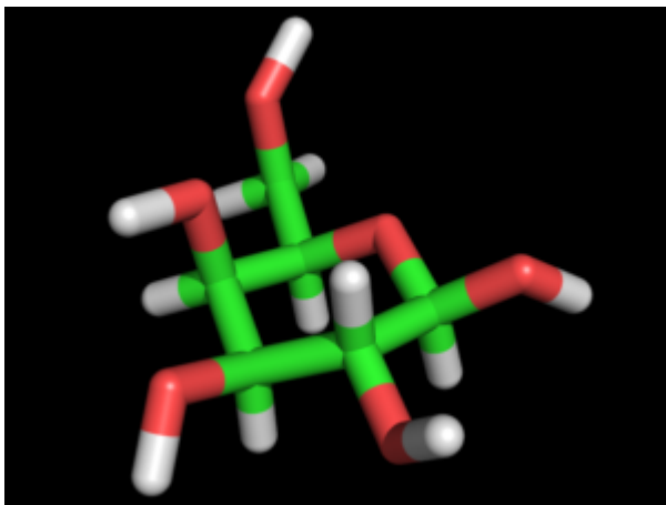
Galactopyranose ?-D
