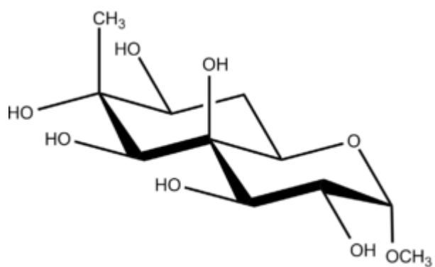
Bradyrhizose
