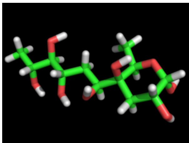
Caryophyllose
