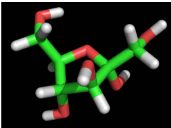
\alpha -D-Fructofuranose
