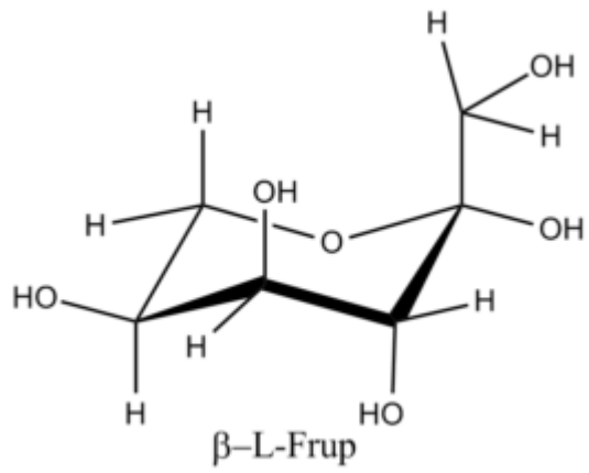
?-L-Fructopyranose
