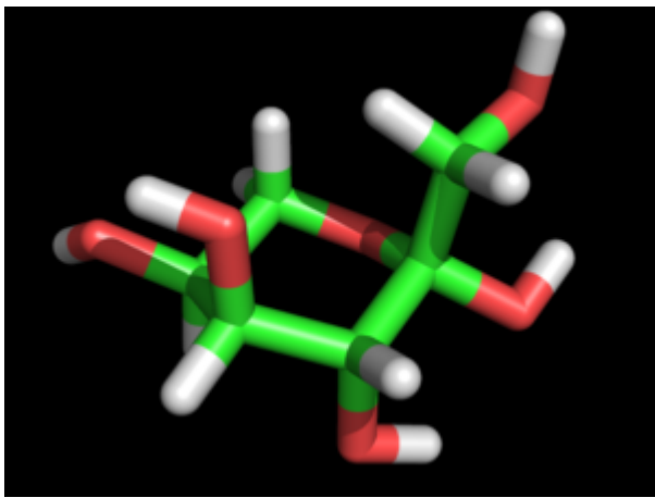
?-L-Fructopyranose
