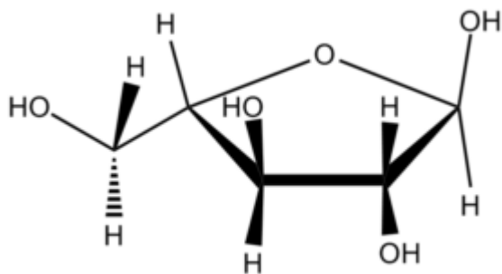
\alpha -L-Xylf
