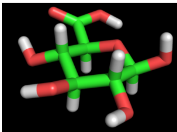
Glucopyranuronic \beta -D
