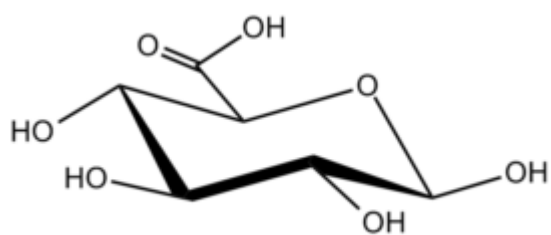
Glucopyranuronic \beta -D
