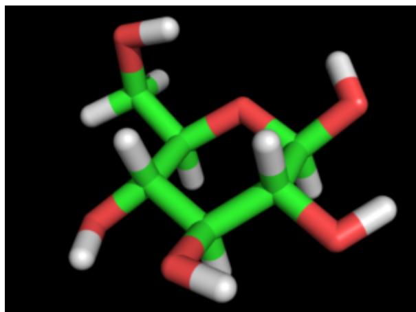
Glucopyranose \beta -D
