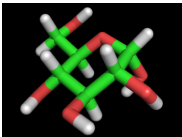
Glucopyranose \alpha -D
