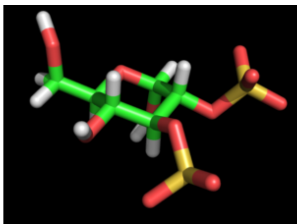
Glucopyranose 2,3-S \hat{\pm} -D
