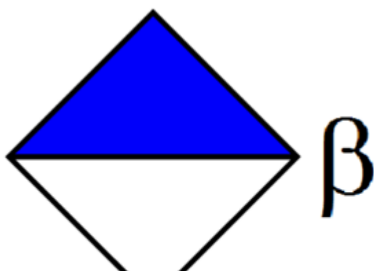
Glucopyranuronic 2-S \beta -D
