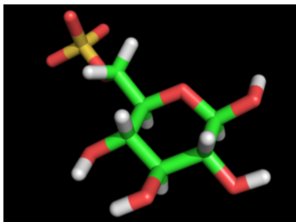
Glucopyranose 6-S \beta -D
