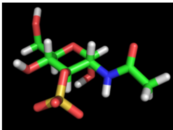
Glucosamine 3-S Î±-D
