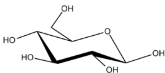
Glucopyranose \beta -D
