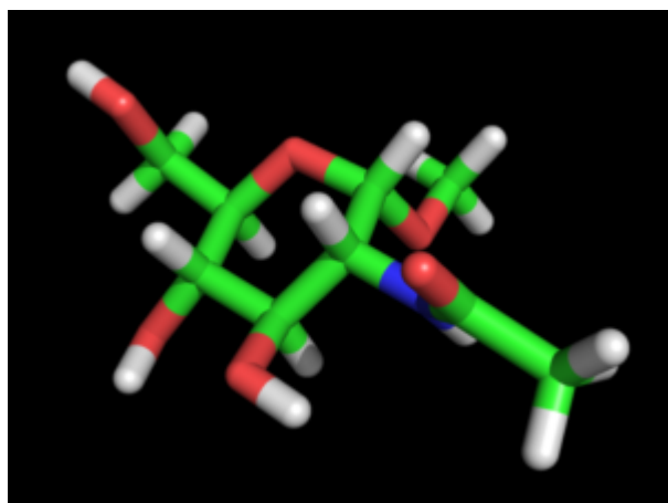
N-Acetyl Glucosamine \alpha -D
