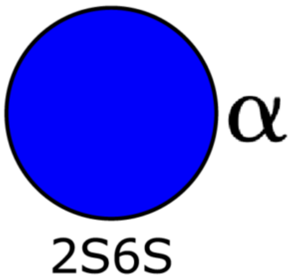
Glucopyranose 2,3-S \alpha -D
