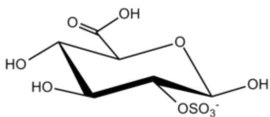
Glucopyranuronic 2-S \beta -D
