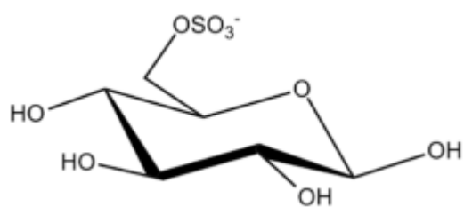
Glucopyranose 6-S \beta -D
