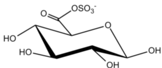
Glucopyranuronic 6-S \beta -D
