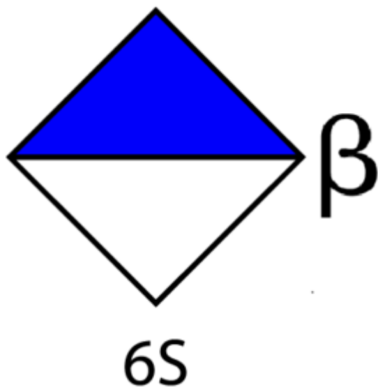
Glucopyranuronic 6-S \beta -D
