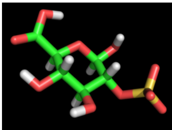
Glucopyranuronic 2-S \beta -D
