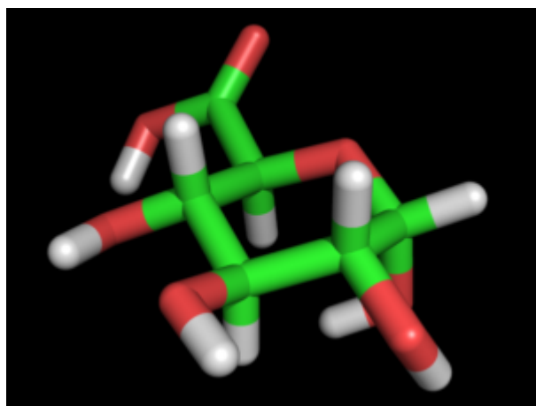
Glucopyranuronic \hat{1}\pm -D
