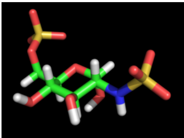
Glucosamine 6-S Î±-D
