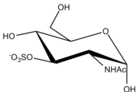
Glucosamine 3-S Î±-D
