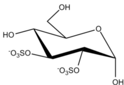
Glucopyranose 2,3-S \hat{\pm} -D
