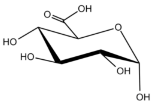
Glucopyranuronic \hat{1}\pm -D
