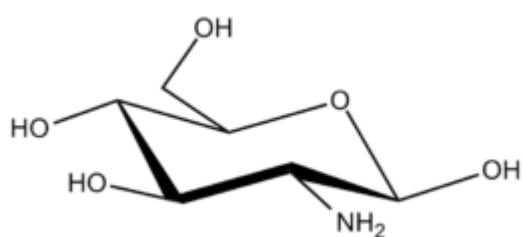
Glucosamine \beta -D
