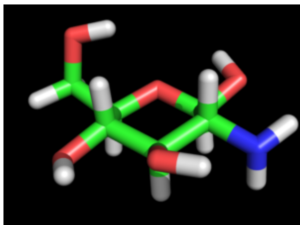
Glucosamine \beta -D
