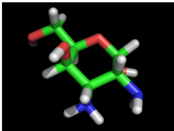
DAG Î±-D : Di-Amino Î±-D Glucose
