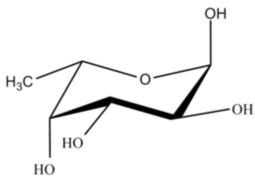
Fucopyranose \alpha -L
