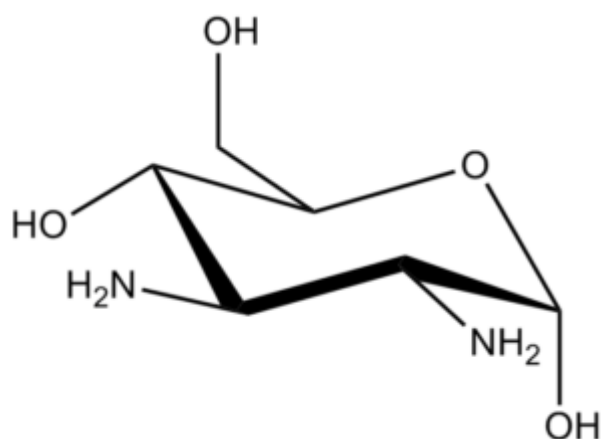
DAG Î±-D : Di-Amino Î±-D Glucose
