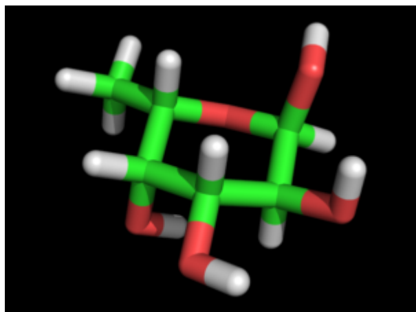
Fucopyranose \alpha -L
