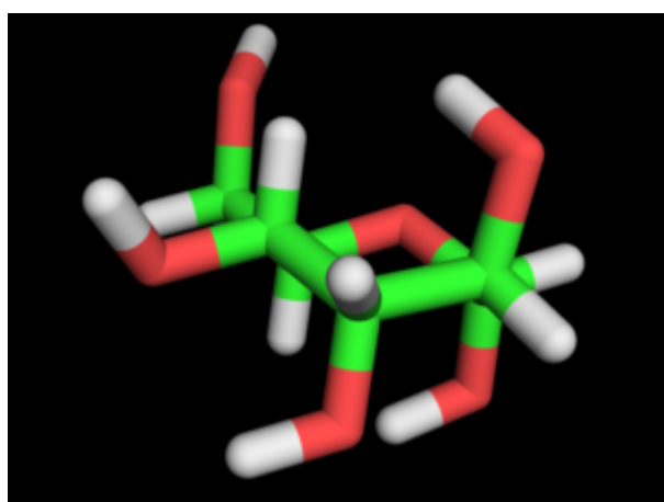
Altro pyranose \hat{1}\pm -D
